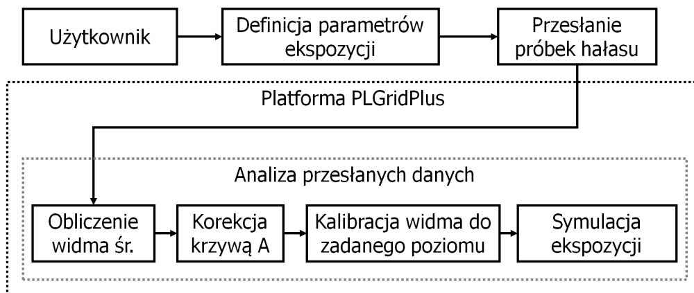
Rys. 2. Schemat działania usługi Słuch
